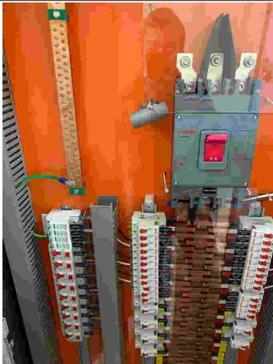
montagem dos quadros TTA
