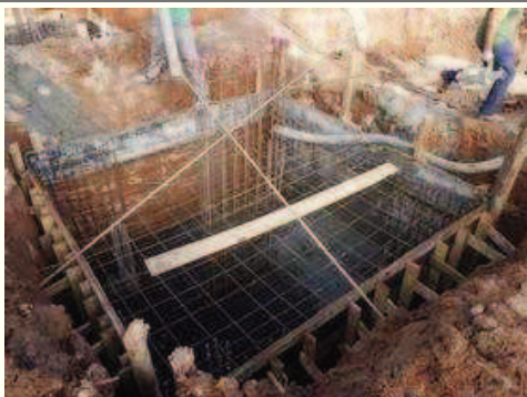
Concretagem
