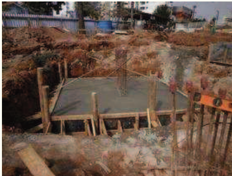
Concretagem 31/07/2015 - Blocos
