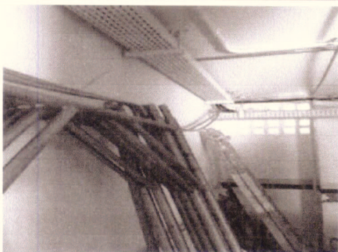
Passagem de fiação 120mm 2 para ligação do Quadro Nobreak
