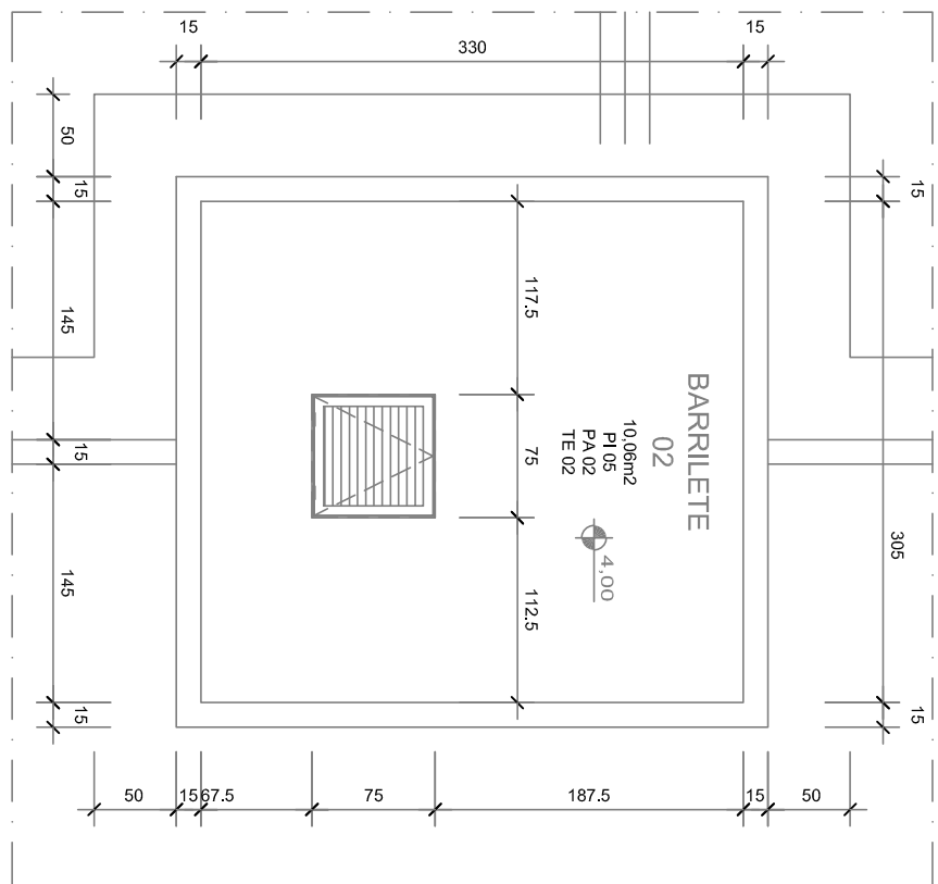
Planta do Barrilete 02 Escala : 1/50
