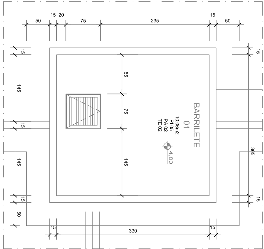
Planta do Barrilete 01 Escala : 1/50
